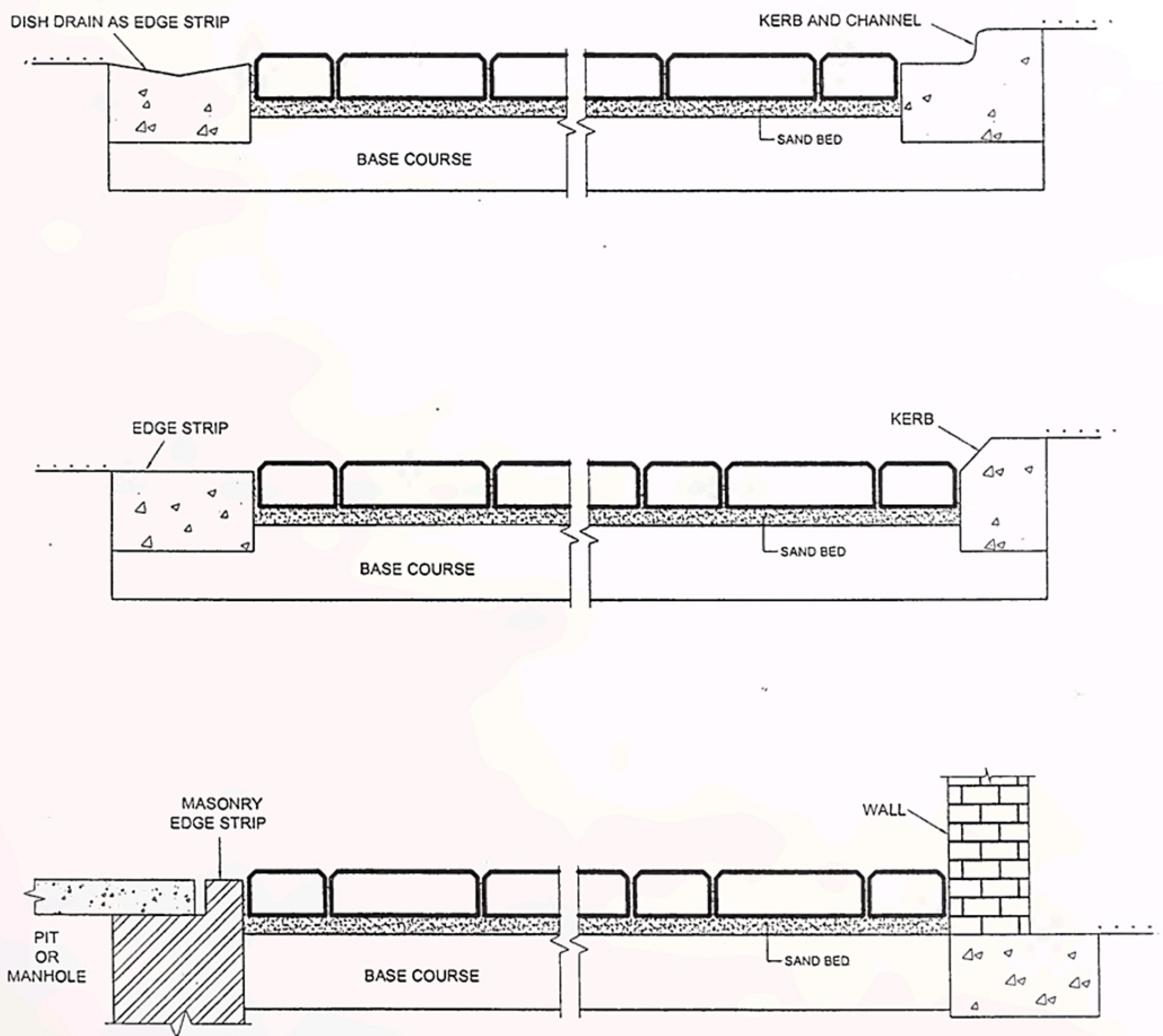
Fig. 8. Edge restraints
