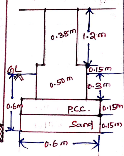
(Wall foundation)
