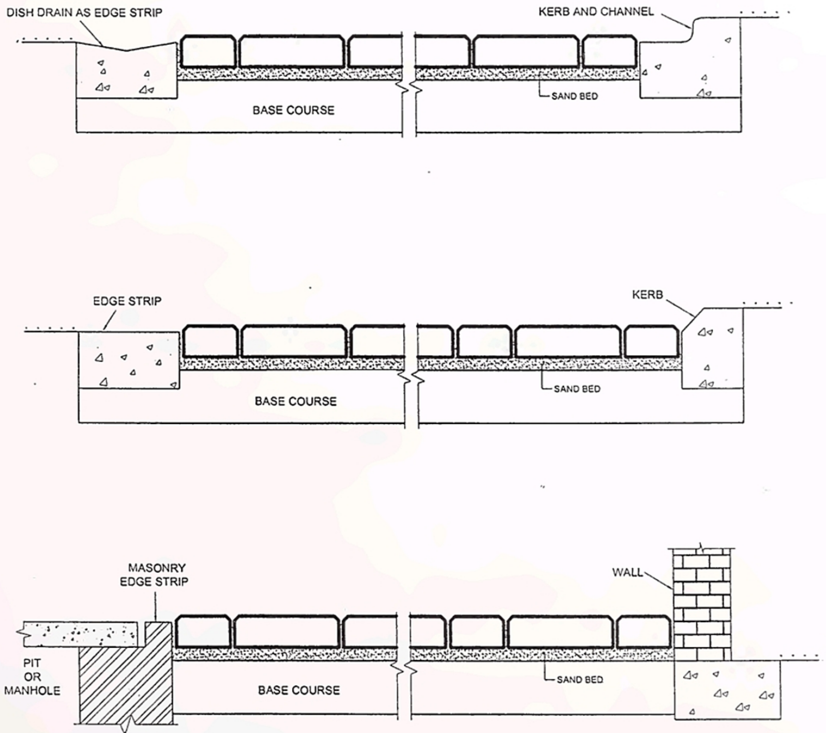
Fig. 8. Edge restraints
